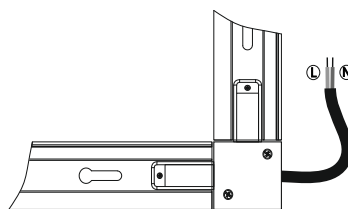
Коннектор угловой с вводом питания
