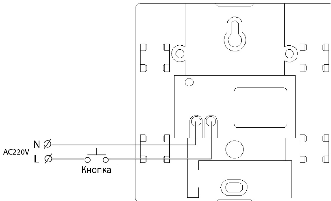
Схема подключения
